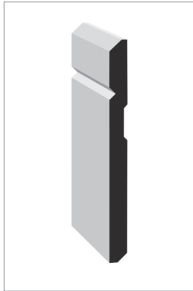
T-8283 1/2" x 6"
